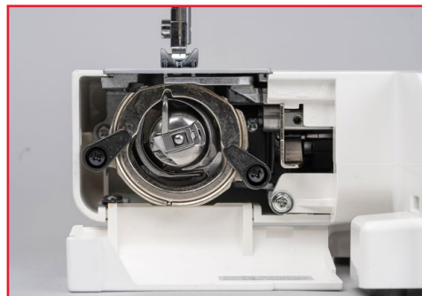
Crochet oscillant vertical à chargement frontal
