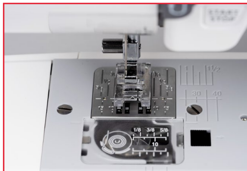
Crochet rotatif horizontal
