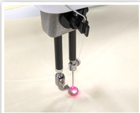
PART: HG01005-JA
