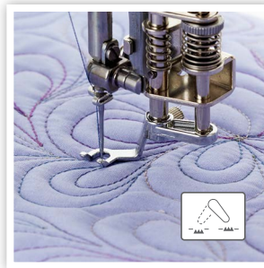
LEVIER DES GRIFFES D'ENTRAÎNEMENT : PIQUAGE EN MOUVEMENT LIBRE
